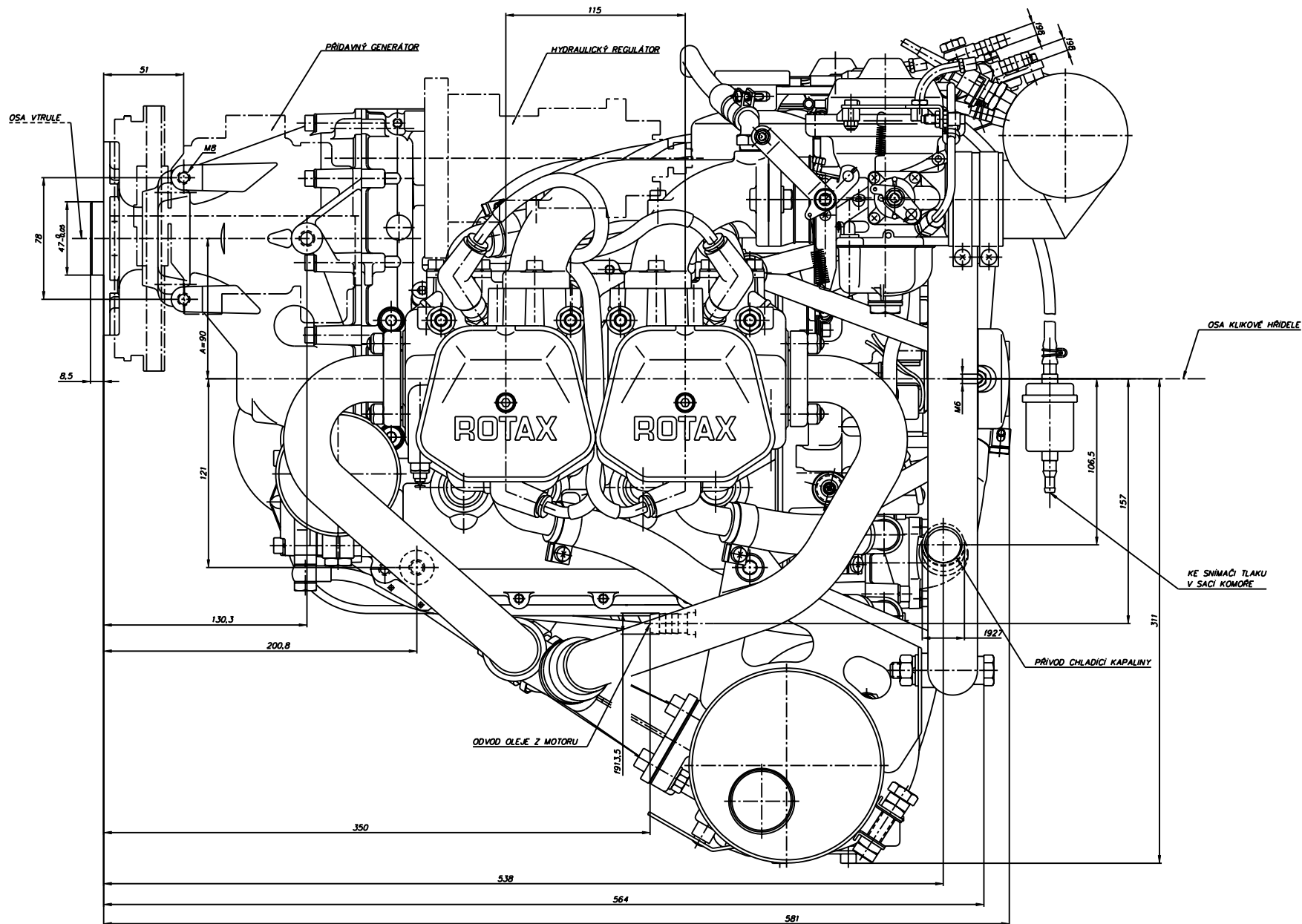
ROTAX 914 UL DCDI – POHLED Z BOKU 914b.dxf
