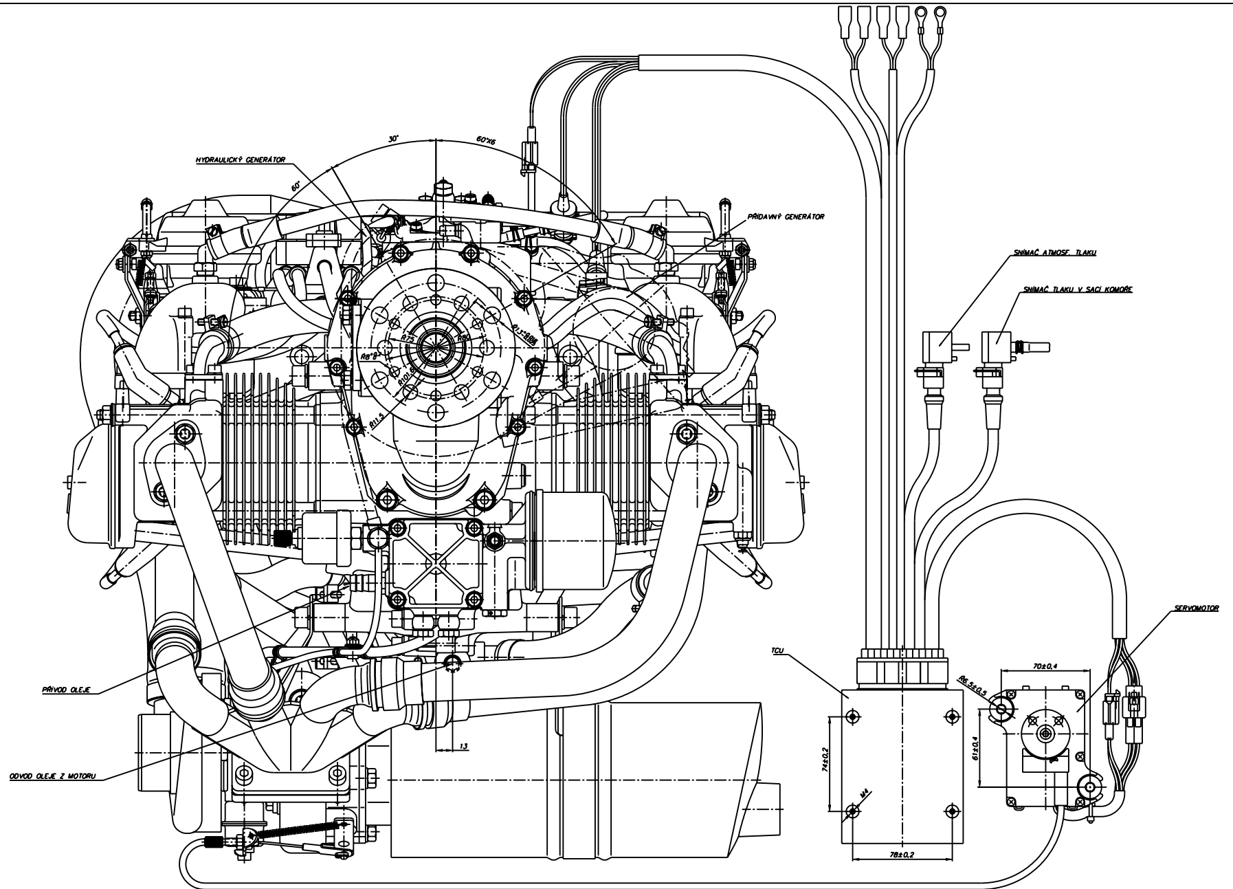
ROTAX 914 UL DCDI – POHLED OD VRTULE 914v.dxf " pouze pro informaci "
