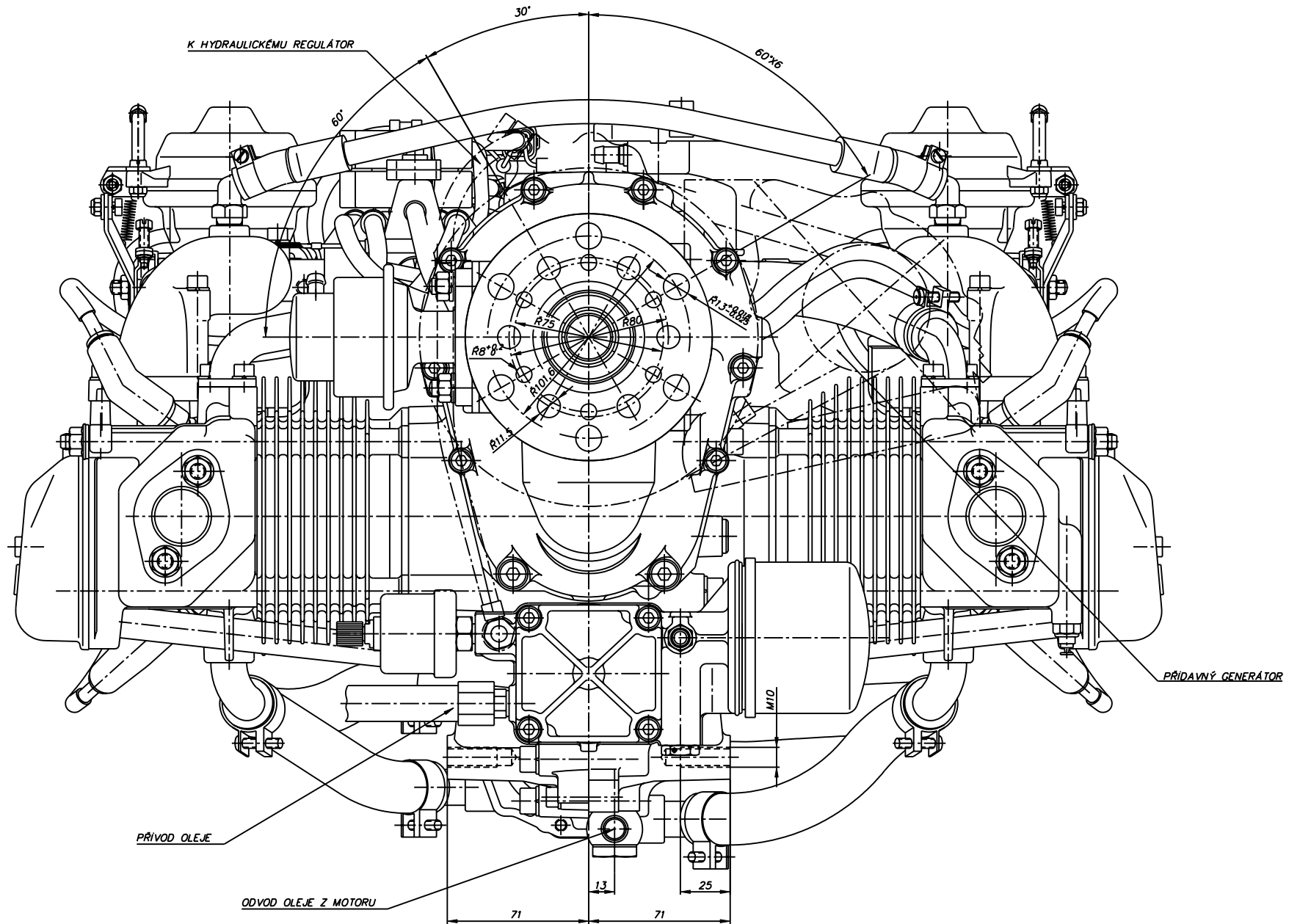
ROTAX 912 UL DCDI – POHLED OD VRTULE 912v.dxf
